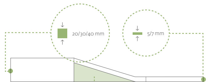
Transition Reducer / Rampa de transición
